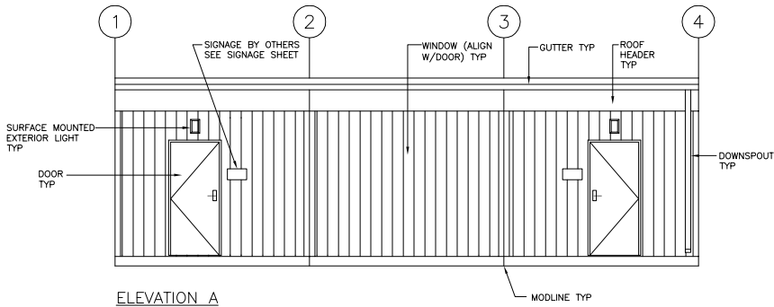
ELEVATION A
